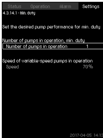
Fig. 92 Min. duty
