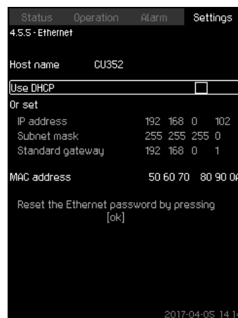
Fig. 127 Ethernet
