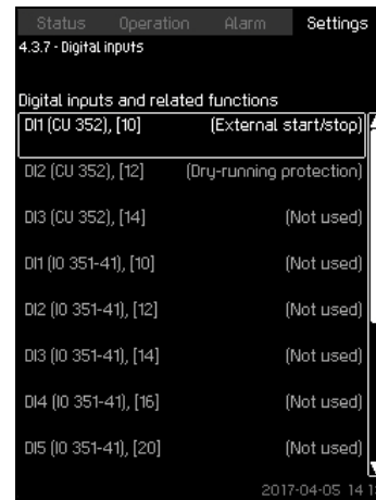
Fig. 81 Digital inputs
