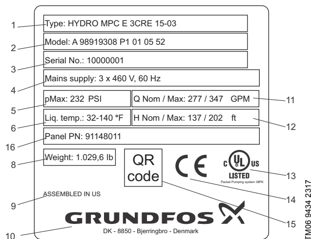
Fig. 10 Nameplate
